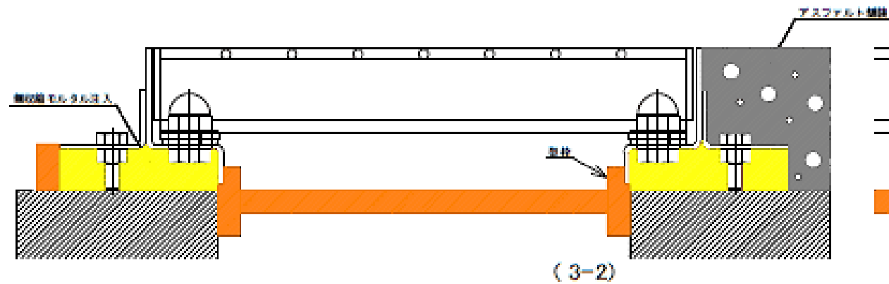
A-A'断面 型枠取付・モルタル注入・アスファルト舗装施工図
