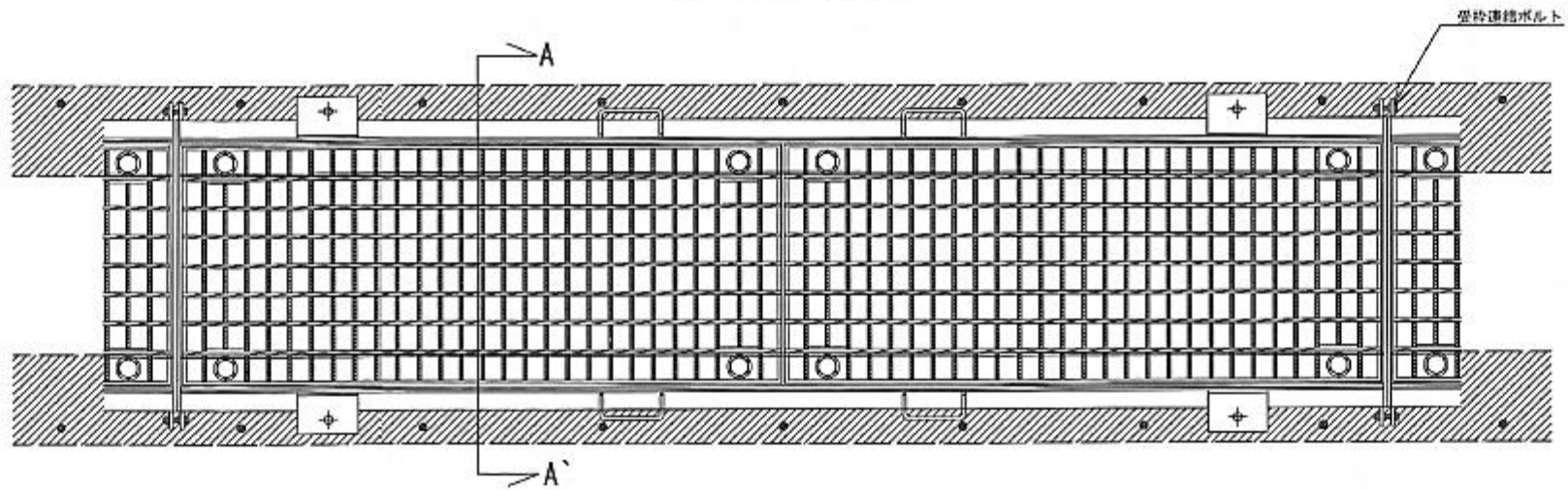
型枠・本体設置平面図
